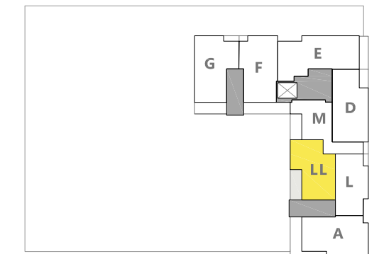
PLANTA TIPO (DE 1ª-5ª-6ª A 8ª)
